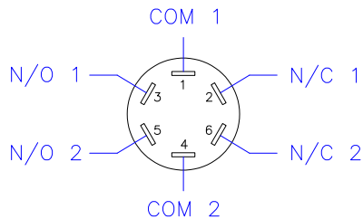
WIRING
